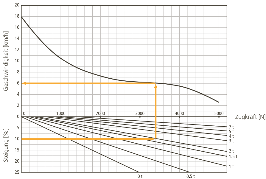
Leistungsschaubild EZS 570
